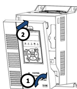
Рис.2-7 Снятие пластикового корпуса
