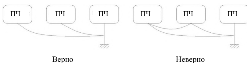
Рис. 3-5 Заземление
